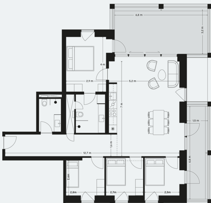
Lejlighedsplan
