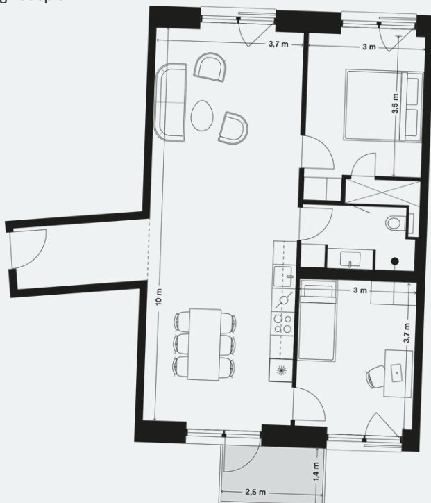
Lejlighedsplan
