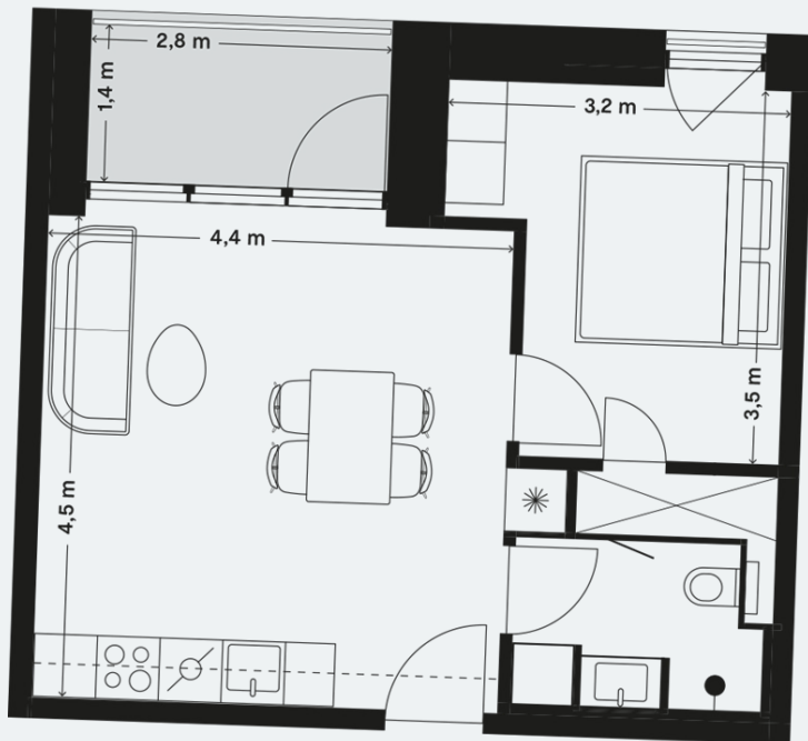
Lejlighedsplan
