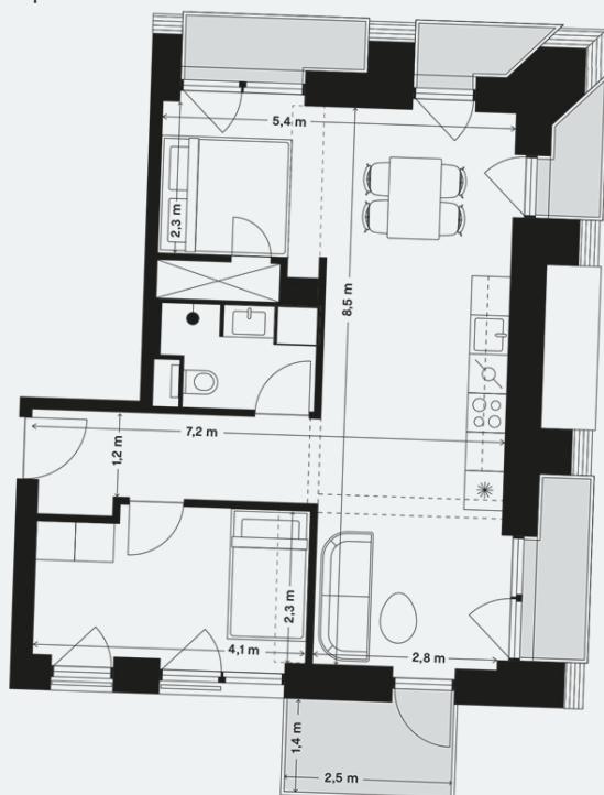
Lejlighedsplan
